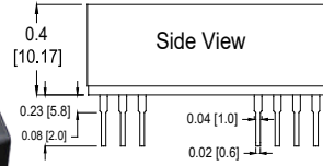
ESAS Series DIP24 Metal Case / Plastic Case
