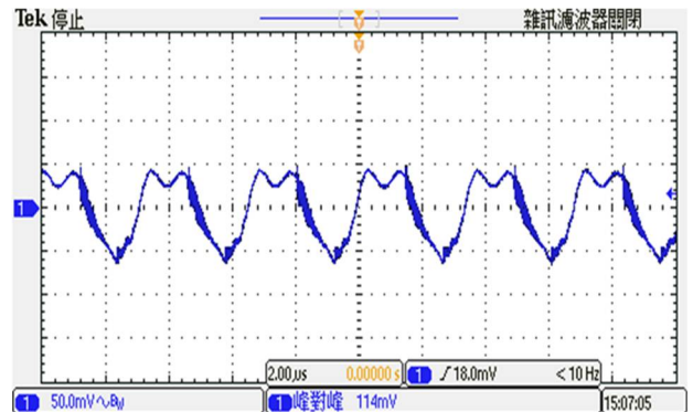
图 8: 出输出电压纹波与噪声(满载). (典型输入, 于输出端加 1 \mu F MLCC 陶瓷电容)
