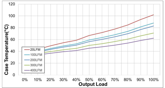
图 4: 工作壳温 VS 输出负载(满载)
