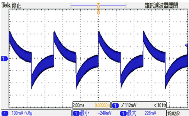
图 7: 进阶负载的输出变化 (典型输入, 于 50~75%的 \Delta I_o/\Delta t = 1A/\mu s 输出电流)
