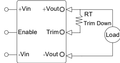
图 2. 电阻调整输出电压示意图(下调)
