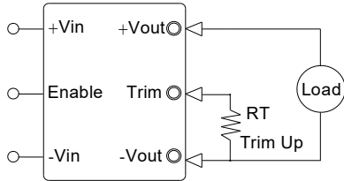
图 1. 电阻调整输出电压示意图(上调)
