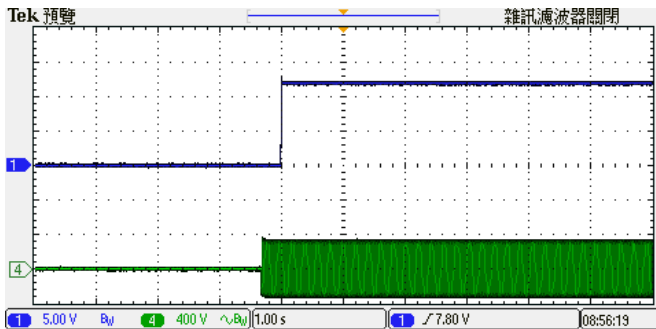
图 3: CH1 = 输出电压, CH4 = 额定输入电压 典型启动波形(满载)
