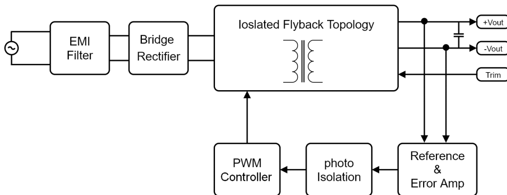
ACE25 系列电路图
