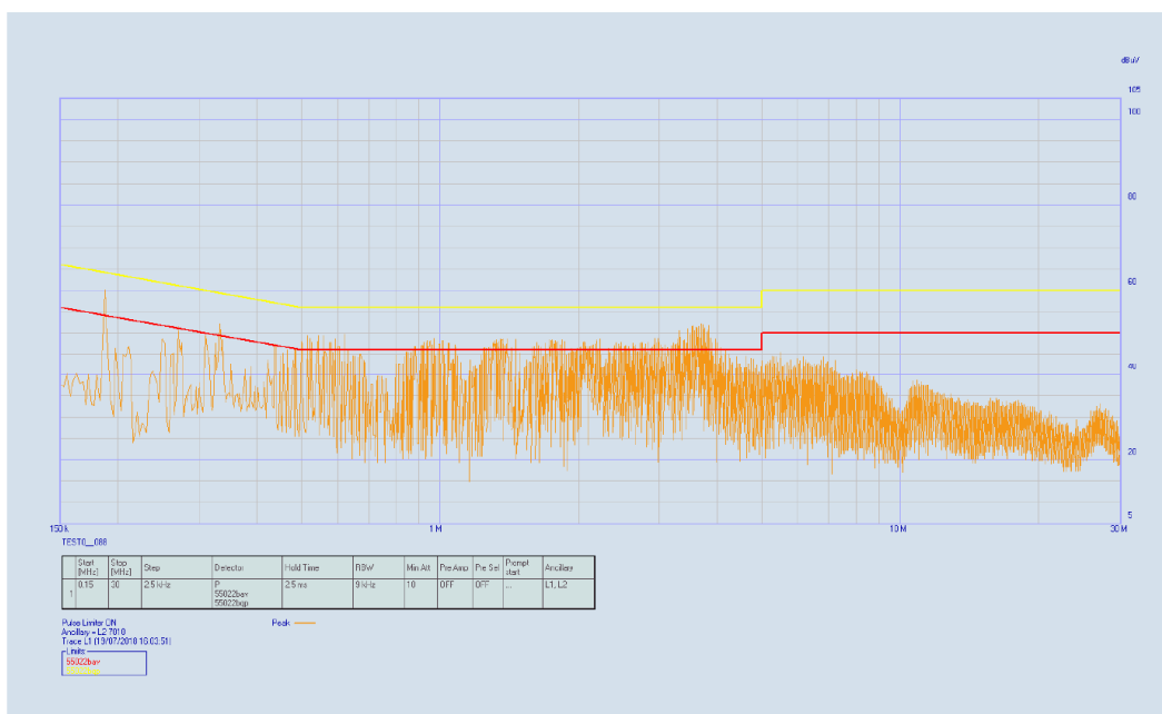
电源模块基础切换带宽 63 kHz.
