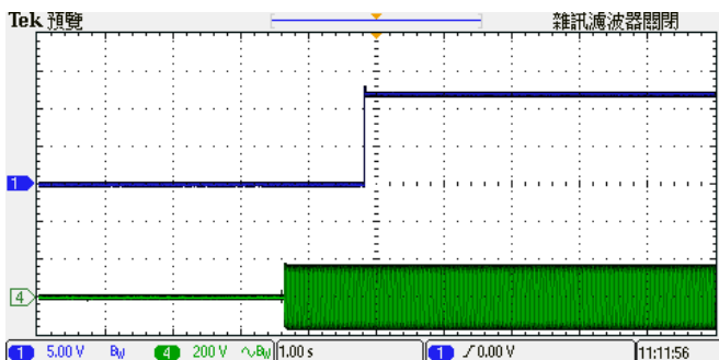
图 5: CH1 = 输出电压, CH4 = 115V 输入电压 启动波形(满载)
