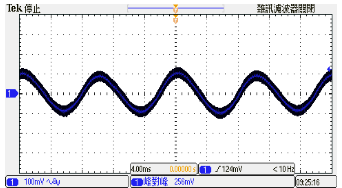
图 6: 输出电压纹波与噪声(满载). (典型输入, 于输出端加 1uF MLCC 陶瓷电容)
