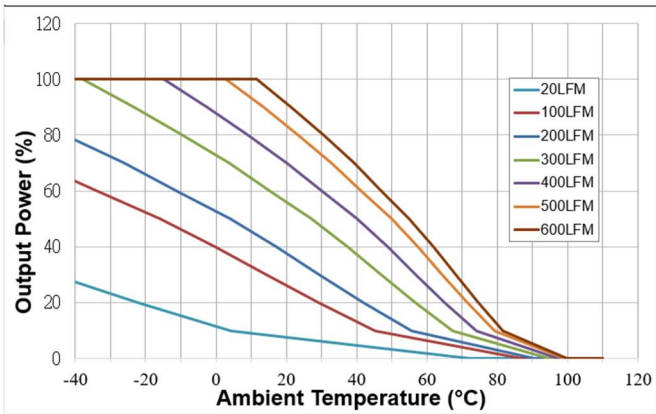
图 3: 环境温度 VS 输出效率额降曲线
