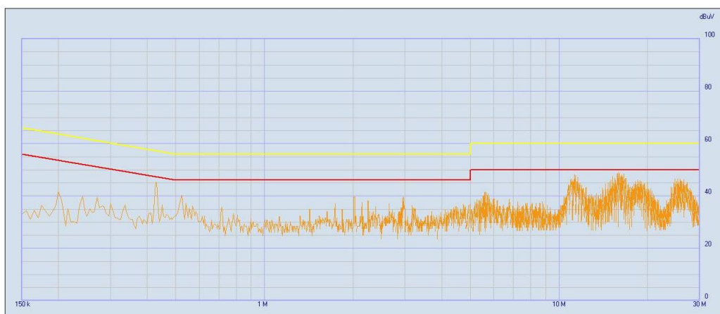
电源模块基础切换带宽 100 kHz.
