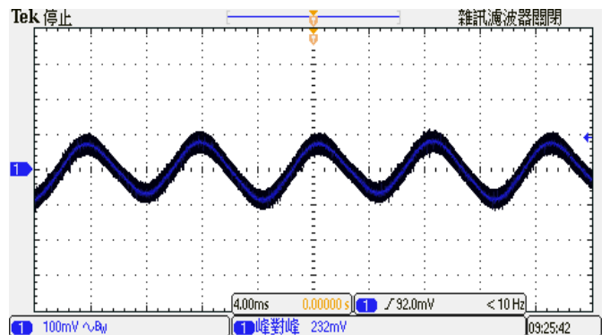
图 8: 输出电压纹波与噪声(满载). (输入电压: 115V, 于输出端加 1uF MLCC 陶瓷电容)
