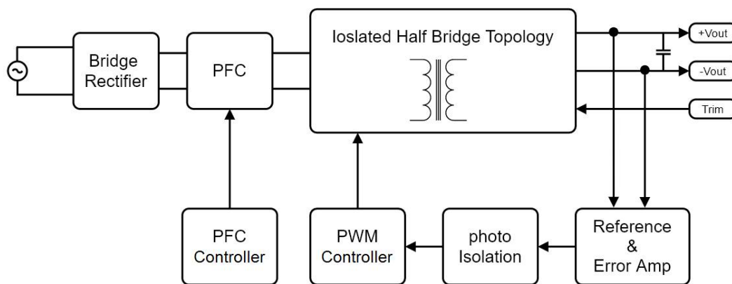
ACH250 系列电路图
