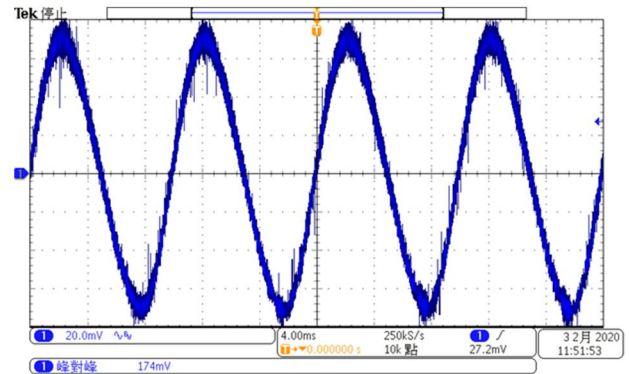
图 6: 输出电压纹波与噪声(满载). (典型输入, 于输出端加 1uF MLCC 陶瓷电容)
