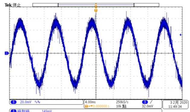
图 8: 输出电压纹波与噪声(满载). (输入电压: 115V, 于输出端加 1uF MLCC 陶瓷电容)
