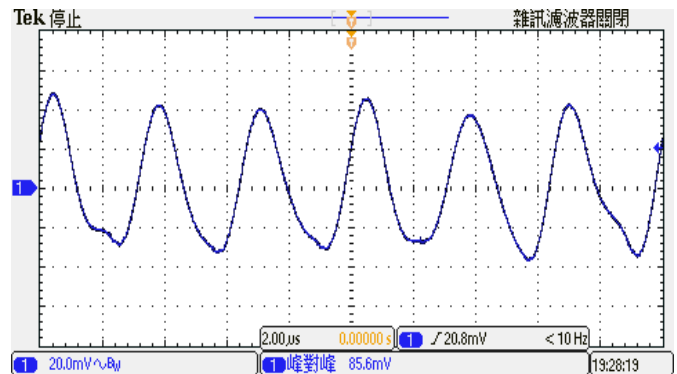
图 8: 出输出电压纹波与噪声(满载). (典型输入, 于输出端加 1uF MLCC 陶磁电容)
