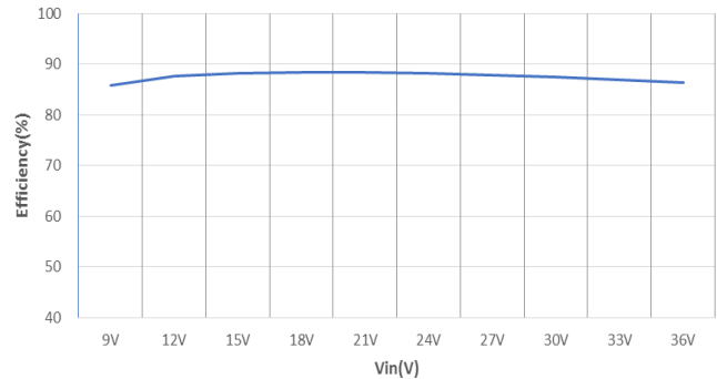
图 2: 效率值 VS 输入电压(满载)
