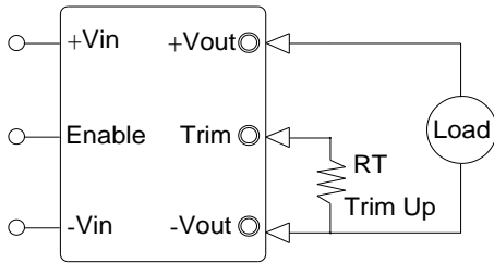
图 1. 电阻调整输出电压示意图(上调)
