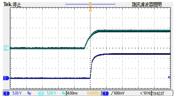
图 6: CH1 = 输出电压, CH3 = 远程摇控电压 典型启动波型(已设定输入电压)
