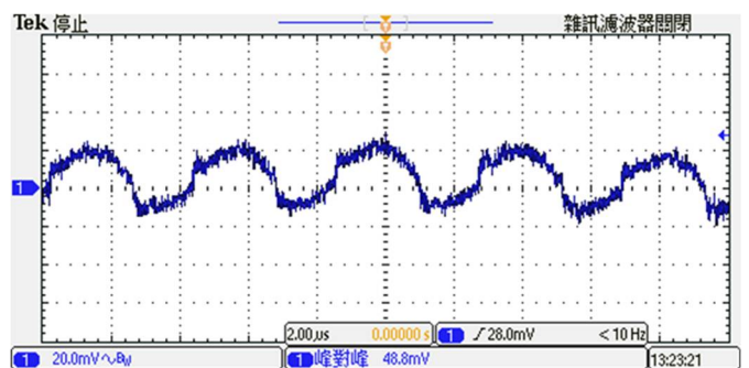
图 8: 输出电压纹波与噪声(满载). (典型输入, 于输出端加 1 \mu F MLCC 陶瓷电容)
