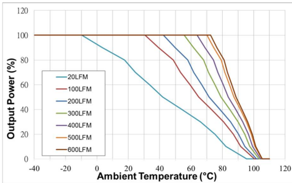
图 3: 环境温度 VS 输出效率降额曲线
