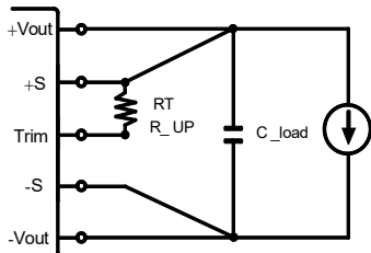
图 1. 电阻调整输出电压示意图(上调)
