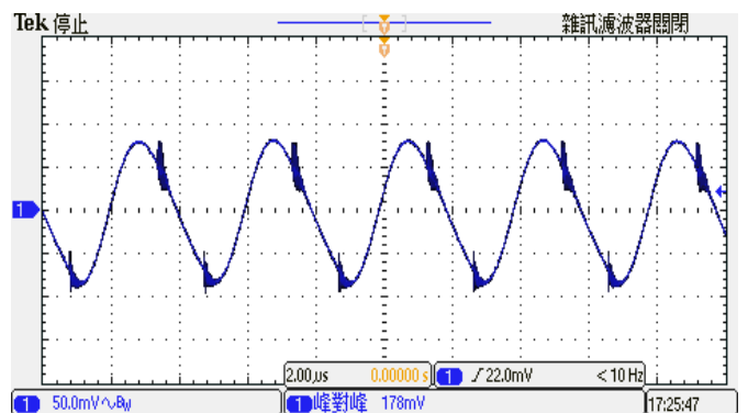
图 8: 输出电压纹波与噪声(满载) (典型输入, 于输出端加 1uF MLCC 陶瓷电容)
