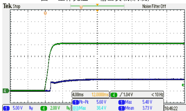
图 6: CH1 = 输出电压, CH3 = 远程遥控电压 典型启动波型(已设定输入电压)
