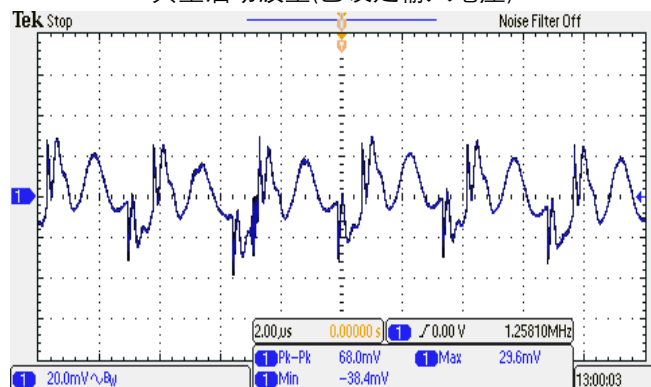
图 8: 输出电压纹波与噪声(满载). (典型输入, 于输出端加 1uF MLCC 陶瓷电容)
