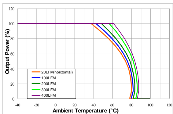
图 3: 环境温度 VS 输出效率额降曲线
