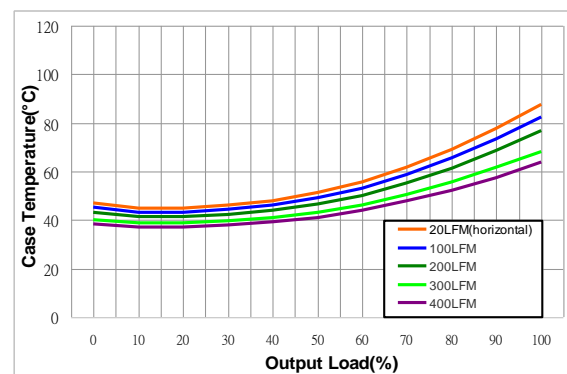
图 4: 工作壳温 VS 输出负载(满载)
