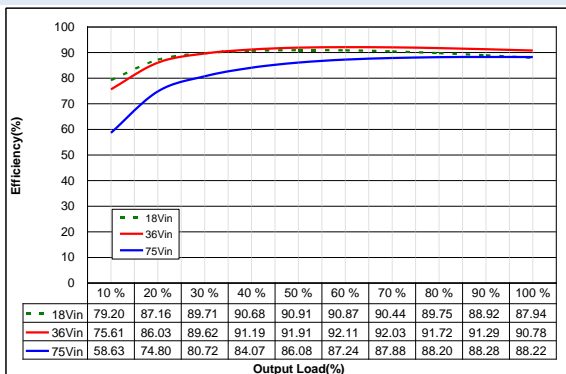
图 1: 效率值 VS 输出负载 分别于最小、额定、最大输出电压时
