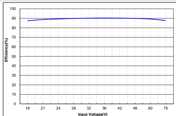
图 2: 效率值 VS 输入电压(满载)
