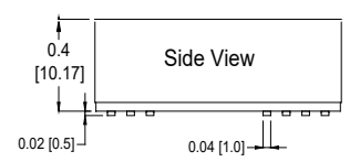
ESAS Series SMD24 Metal Case / Plastic Case
