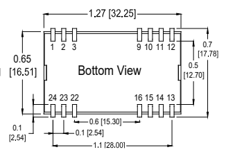
ESAS Series SMD 24 Pinout
