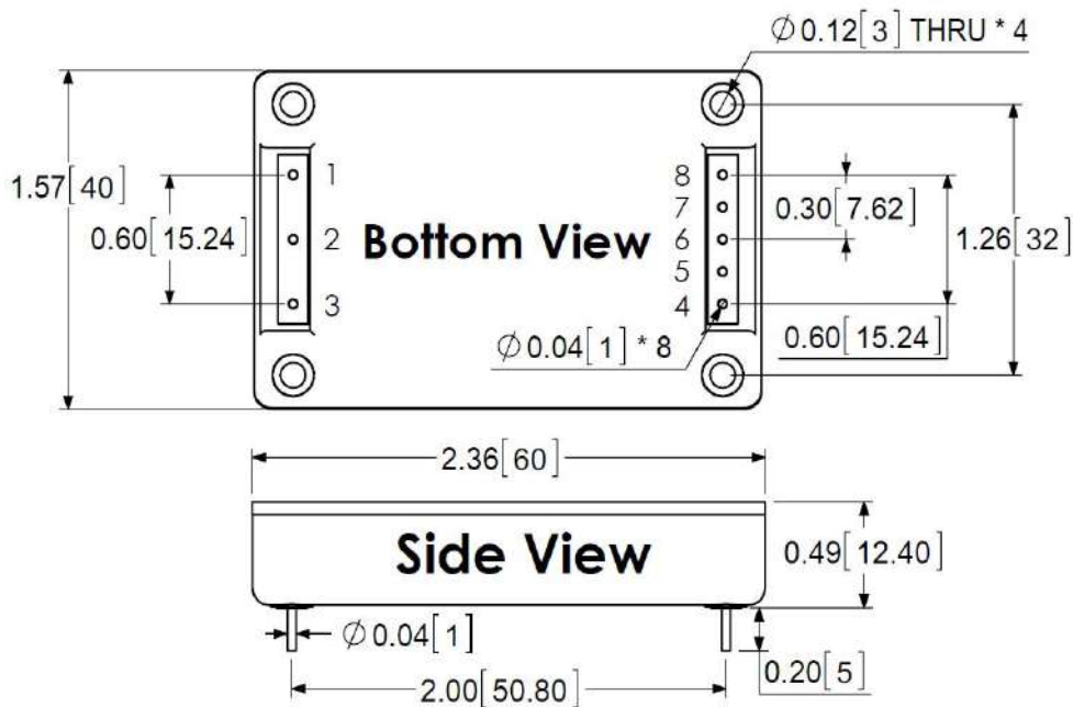
尺寸图 - B
