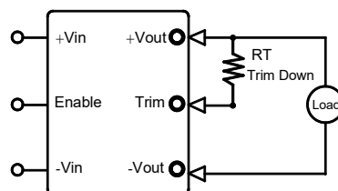
图 2. 电阻调整输出电压示意图(下调)
